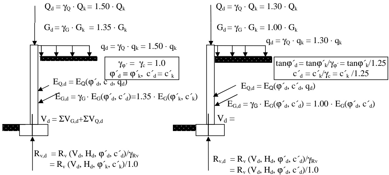
a) DA 1: Combination 1
